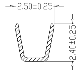
SEC:A-A
